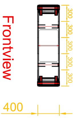
5 X HEB-400
